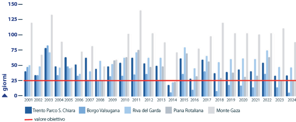
Figura 5.16: O 3 – superamenti del valore obiettivo
