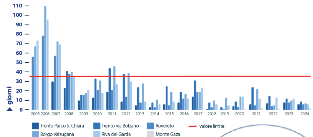
Figura 5.3: PM10 – numero di superamenti del valore limite giornaliero
